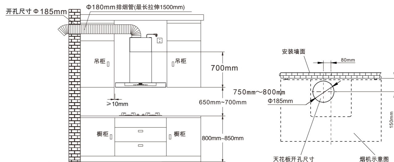
图一 整机与橱柜装配示意图
